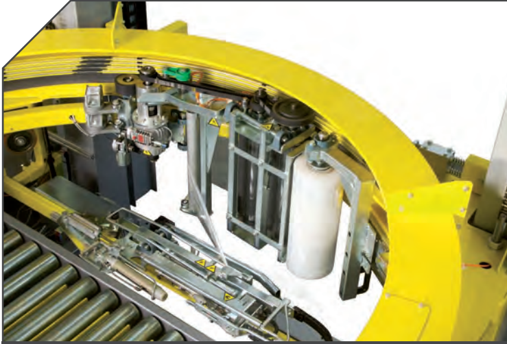
GRUPPO PRESTIRO FILM E GRUPPO PINZA DI TAGLIO FILM (BREVETTATO) FILM PRE-STRETCHING UNIT AND FILM INSERTION CLAMP UNIT (PATENTED) UNIDAD DE PREESTIRADO Y UNIDAD DE PINZA DE CORTE Y INTRODUCCIÓN FILM (PATENTADA) FOLIENVORRECKUNG UND FOLIENEINLEGGZANGE (PATENT)
