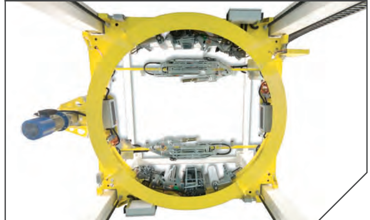
GRUPPO PRESTIRO FILM E GRUPPO PINZA DI TAGLIO FILM (BREVETTATO) FILM PRE-STRETCHING UNIT AND FILM INSERTION CLAMP UNIT (PATENTED) UNIDAD DE PREESTIRADO Y UNIDAD DE PINZA DE CORTE Y INTRODUCCIÓN FILM (PATENTADA) FOLIENVORRECKUNG UND FOLIENEINLEGGZANGE (PATENT)
