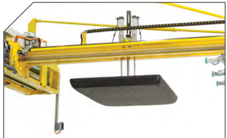
GRUPPO PRESSORE STABILIZZATORE CARICO TOP PRESS PLATE PISON TOP PRESSPLATTE
